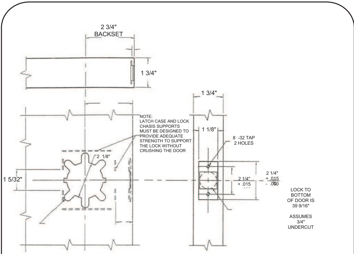
DOOR FACE DETAIL
